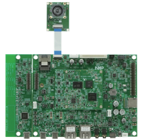
NXP i.MX93 EVK
