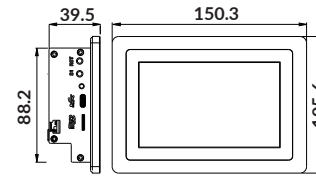
TEP-0500-IMX6UL
